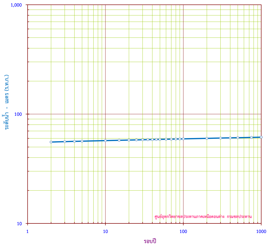
กราฟแสดง ระดับน้ำสูงสุดรายปี ขนาดรอบปีต่างๆ สถานี P.15 อ.คลองขลุง จ.กำแพงเพชร
